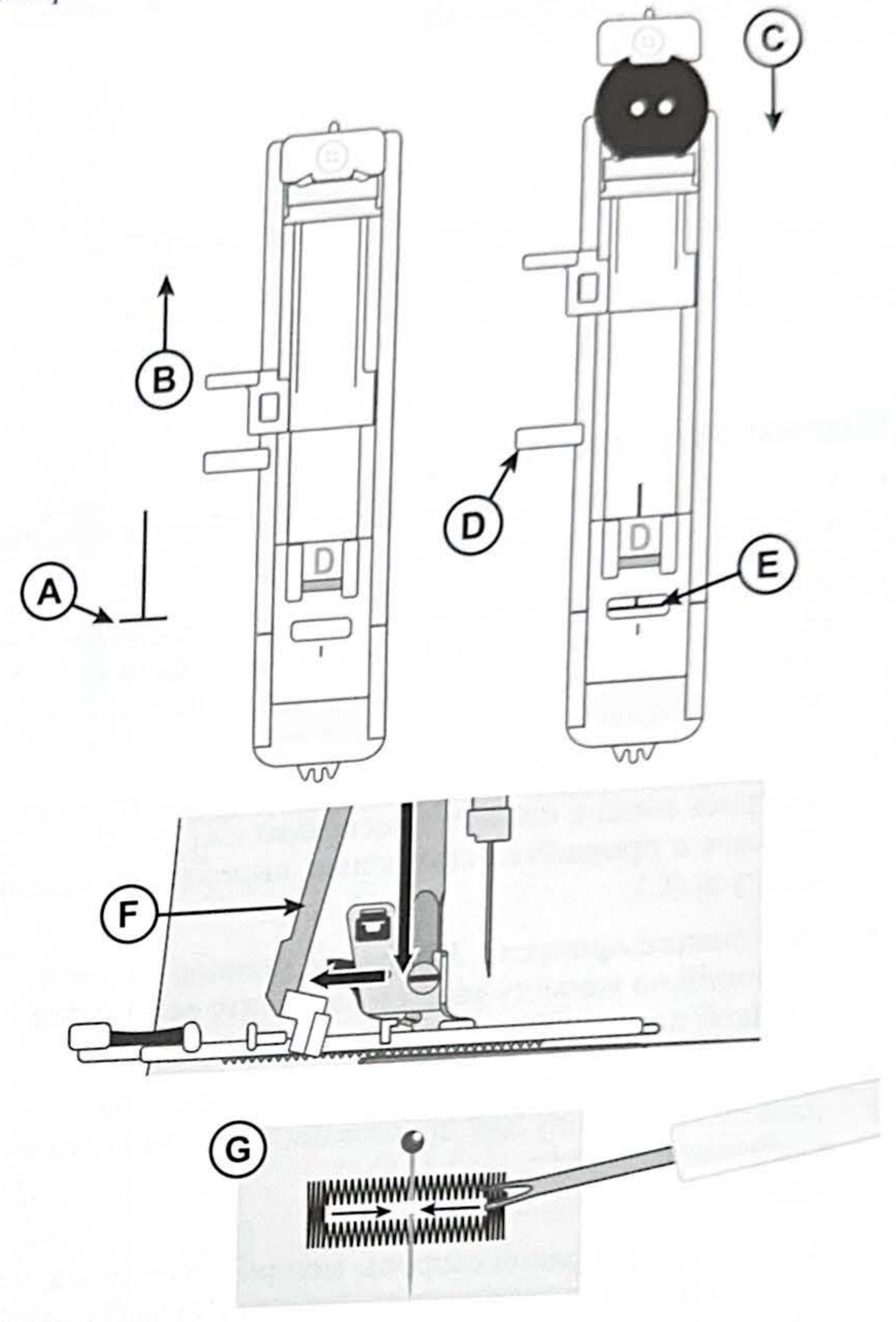
Настройки для петли
