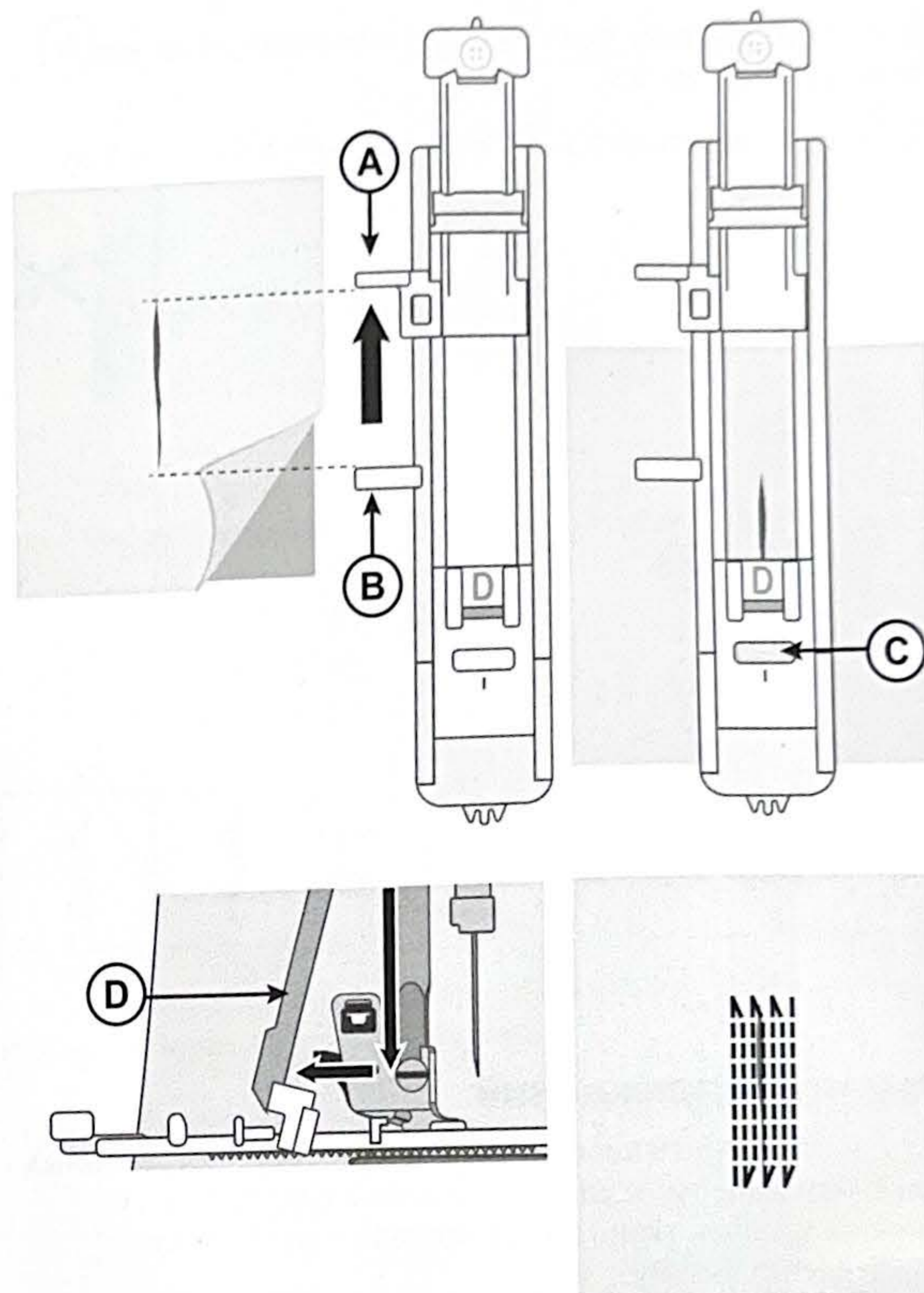
Настройка для штопальной строчки
